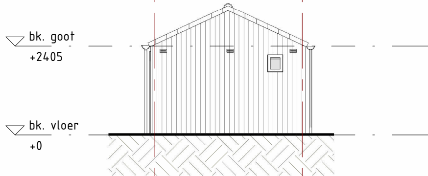
rechtergevel bnr. 52 1 : 100
