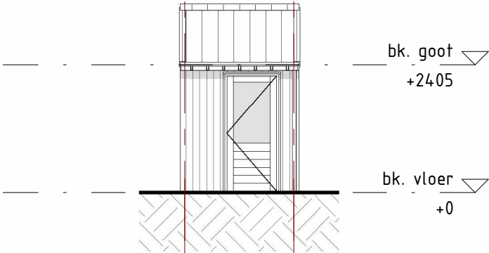
voorgevel 1 : 100
