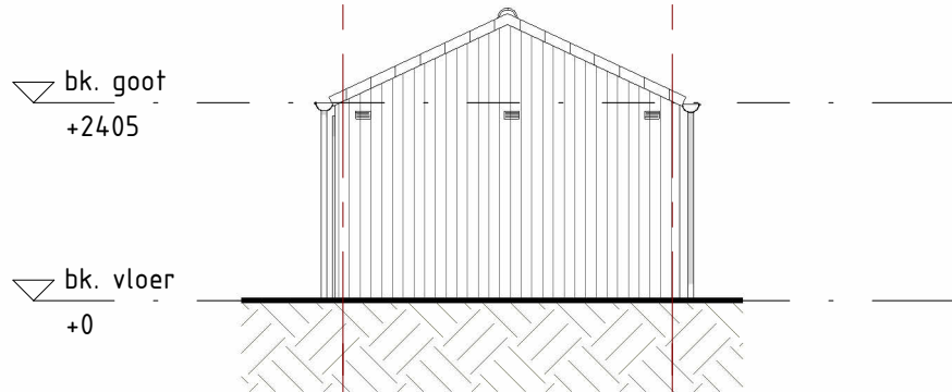
rechtergevel 1 : 100
