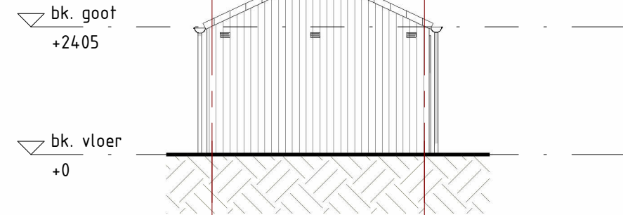
linkergevel 1 : 100
