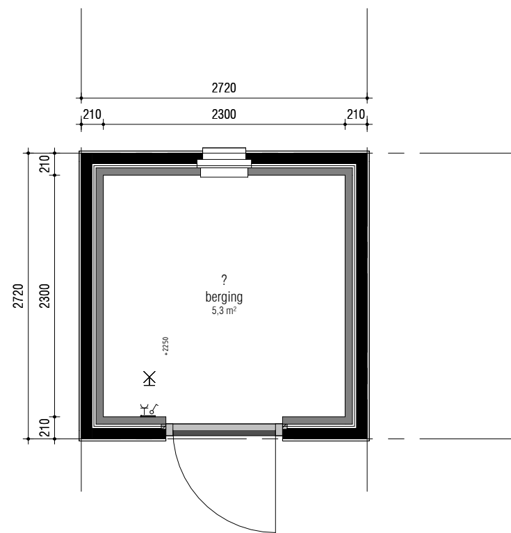
begane grond
