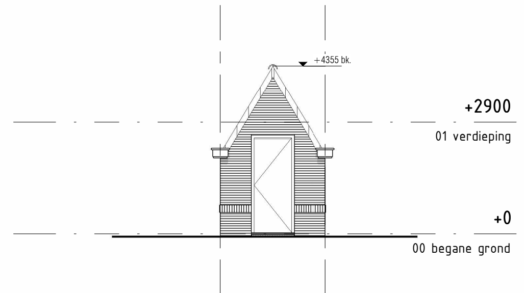
voorgevel
