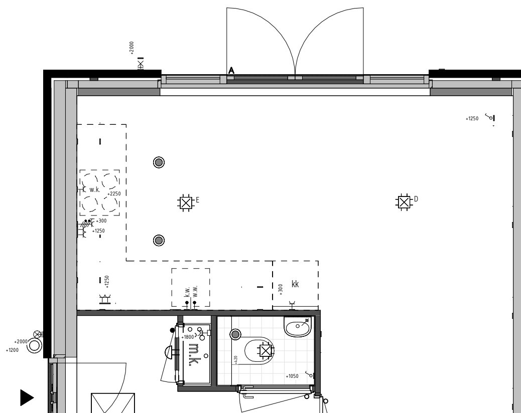
475112 keukenpositie 2 Keukenoptie 2 mogelijk bij bouwnummer: 43
