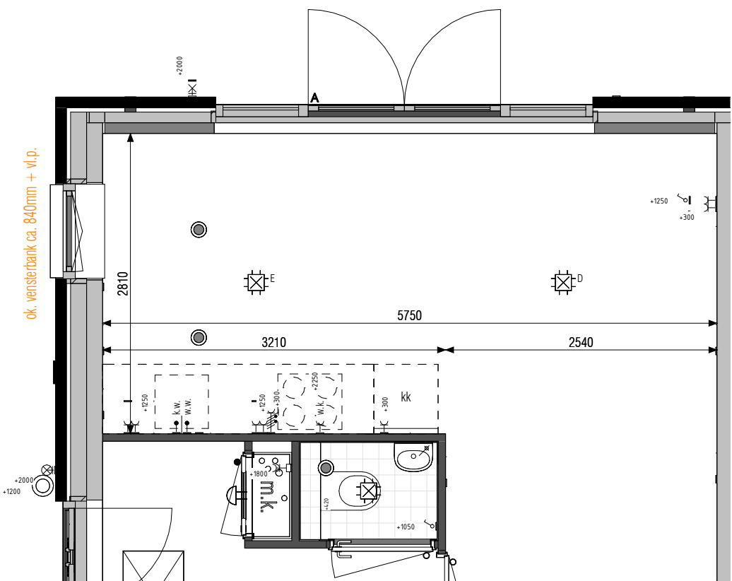
Kopgevel type A bnr: 1 475111 keukenpositie 1 (standaard) Standaard keukenoptie bouwnummer: 1
