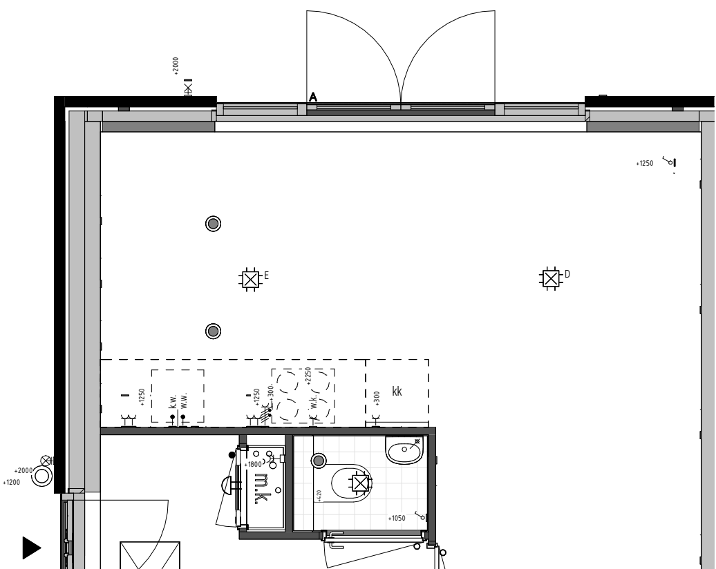
Kopgevel type R bnr: 43 475111 keukenpositie 1 (standaard) Standaard keukenoptie bouwnummer: 43
