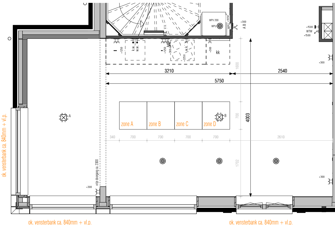
475131 keukenpositie 31 Keukenpositie 31 mogelijk bij bouwnummer: 43
